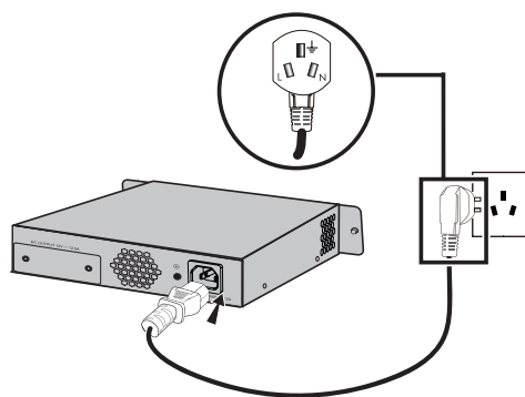
图3-7 TL-RPS150连接电源线示意图
