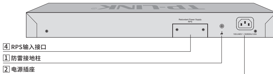
图1-9 TL-SH7428后面板示意图
