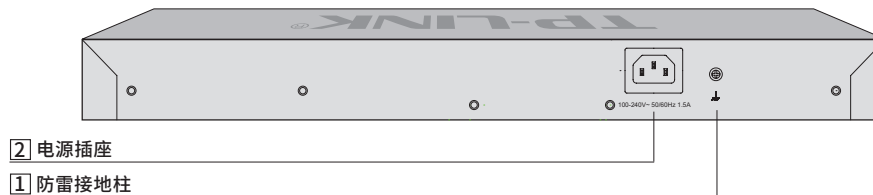
图1-7 TL-SH6428F后面板示意图
