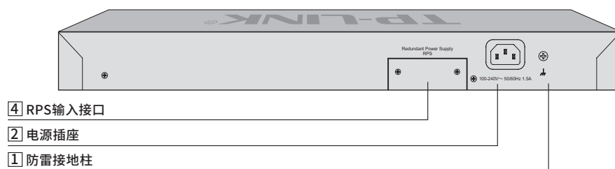
图1-10 TL-SH7428F后面板示意图
