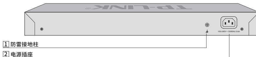
图1-6 TL-SH6428后面板示意图
