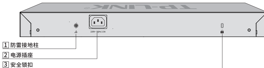
图1-8 TL-SH6428P后面板示意图
