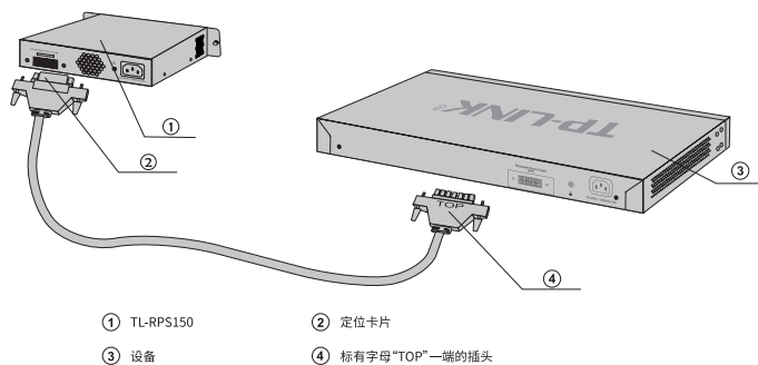
图3-6 连接设备和TL-RPS150示意图
